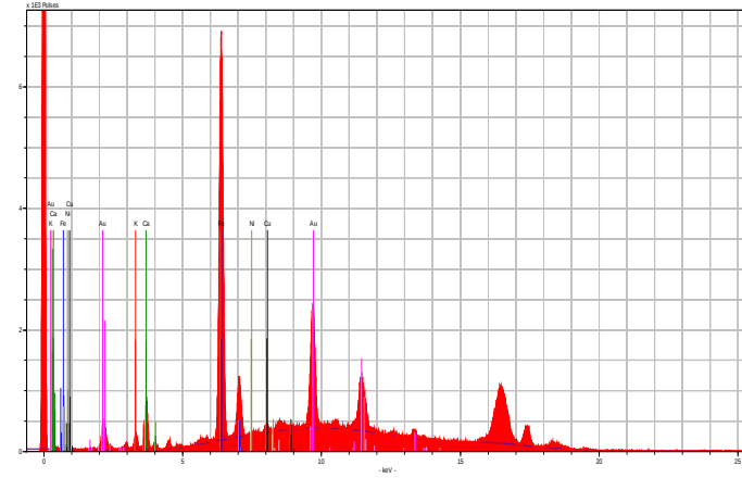
Şekil 2- Miklep şemsesi altın renkli süsleme XRF spektrumu
